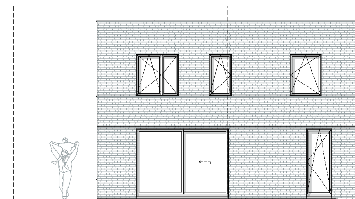
Achtergevel
