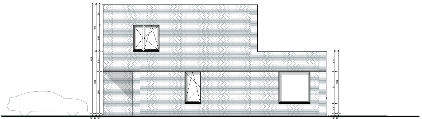
Zijgevel
