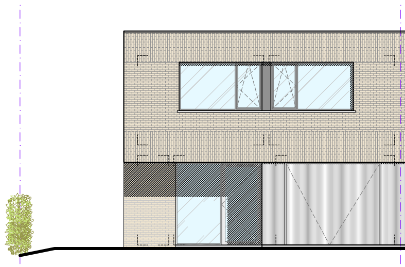
voorgevel
